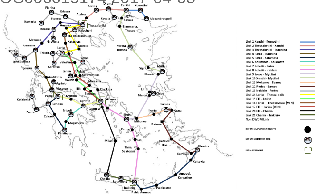
Εικόνα 5 Δίκτυο Οπτικών Ινών ΕΔΕΤ (WAN)
