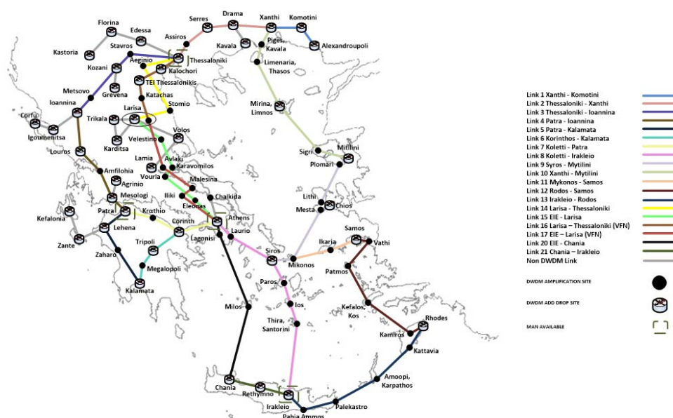
Εικόνα 5 Δίκτυο Οπτικών Ινών ΕΔΕΤ (WAN)
