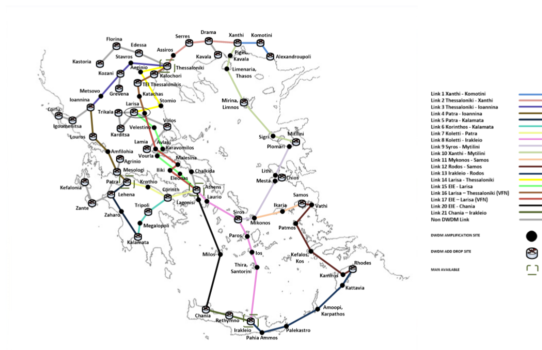
Εικόνα 1 Δίκτυο Οπτικών Ινών ΕΔΕΤ (WAN)
