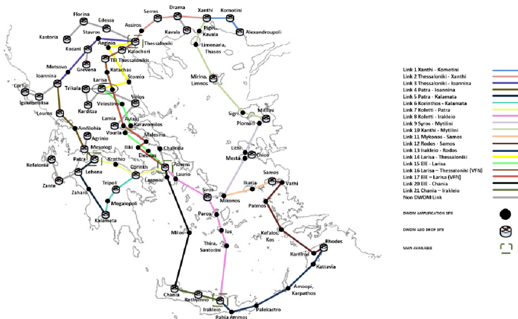
Εικόνα 7 Δίκτυο Οπτικών Ινών ΕΔΥΤΕ (WAN)
