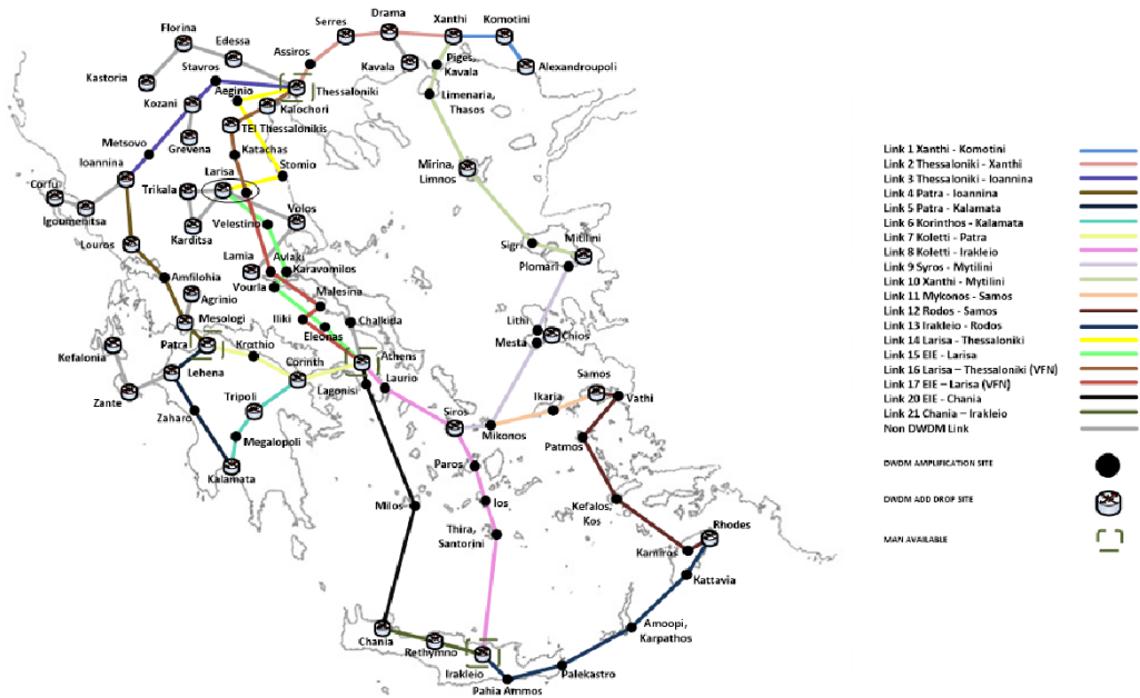
Εικόνα 7 Δίκτυο Οπτικών Ινών ΕΔΥΤ (WAN)
