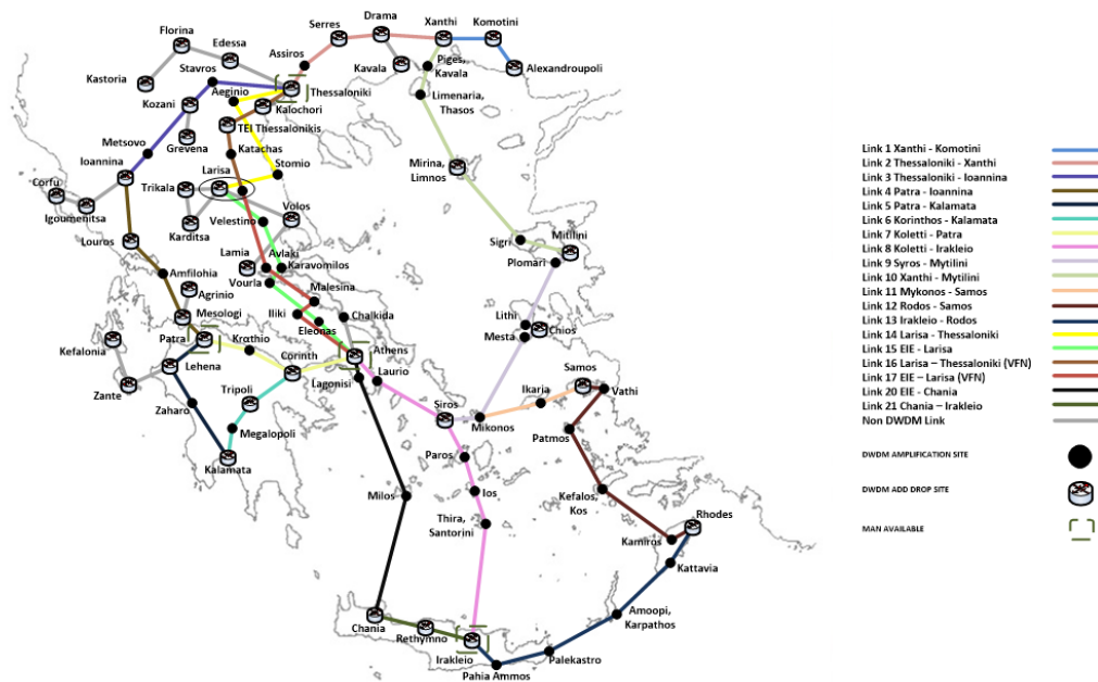
Εικόνα 2 Δίκτυο Οπτικών Ινών ΕΔΕΤ (WAN)
