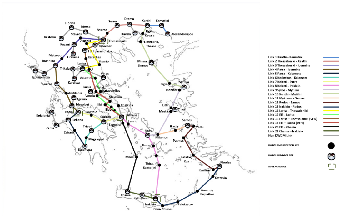
Εικόνα 7 Δίκτυο Οπτικών Ινών ΕΔΥΤ (WAN)
